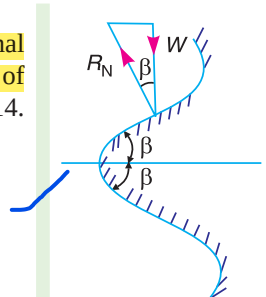
Fig. 10.14. V-thread.
