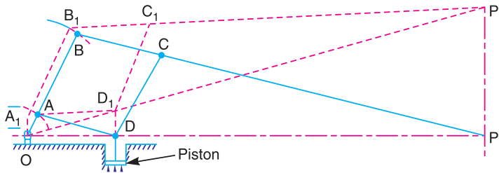
Fig. 9.11. Simplex indicator.
