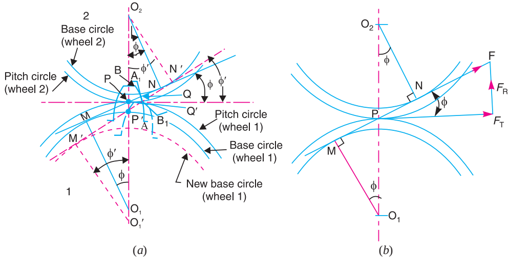
Fig. 12.10. Involute teeth.
